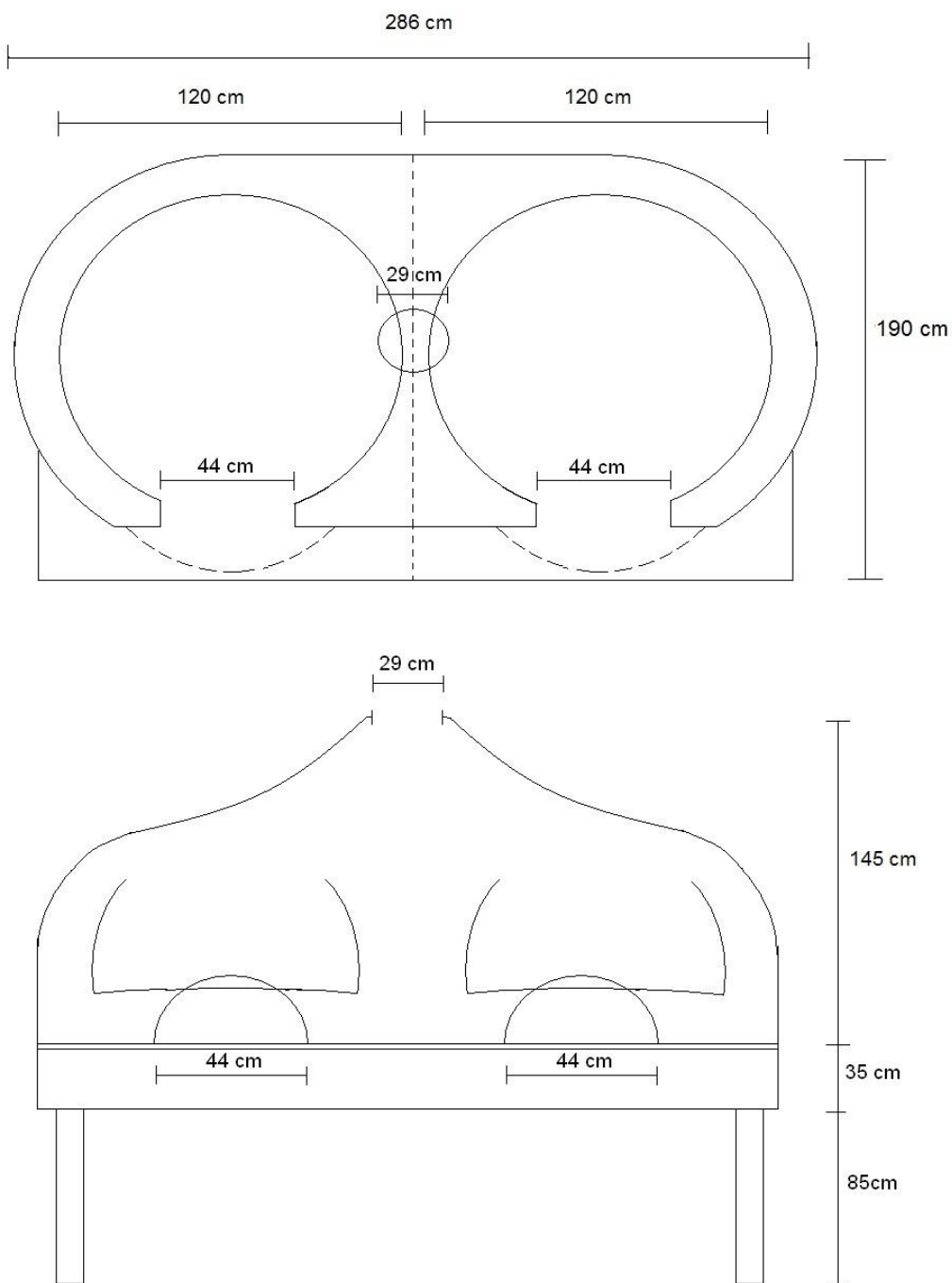
Dimensions of DOPPIO COMBO 5
